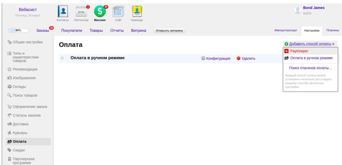
Рисунок 1. Добавление модуля.
