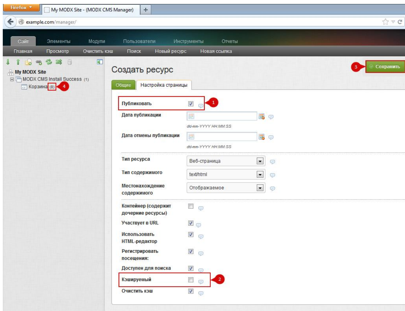
Рисунок 7. Настройка ресурса
