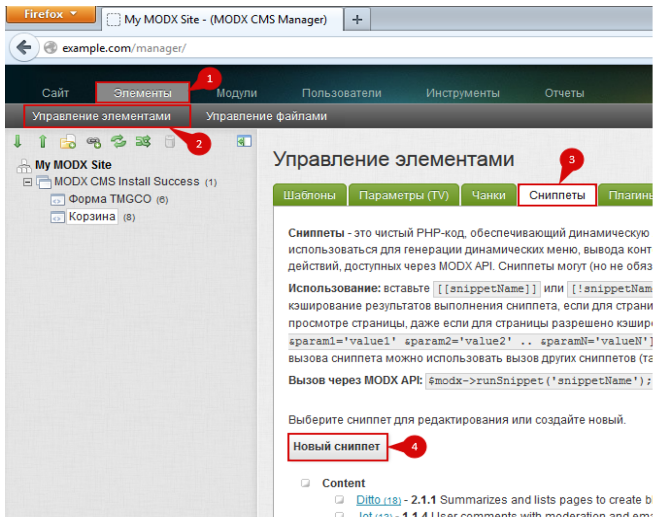
Рисунок 1. Создание сниппета
