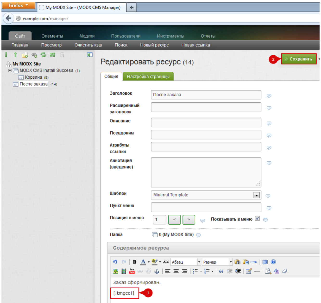
Рисунок 4. Редактирование ресурса
