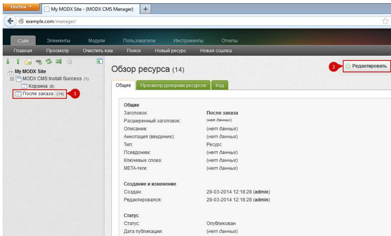
Рисунок 3. Открытие ресурса
