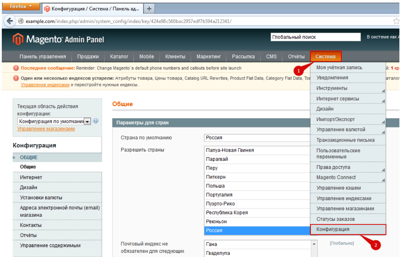
Рисунок 2. Конфигурация Magento
